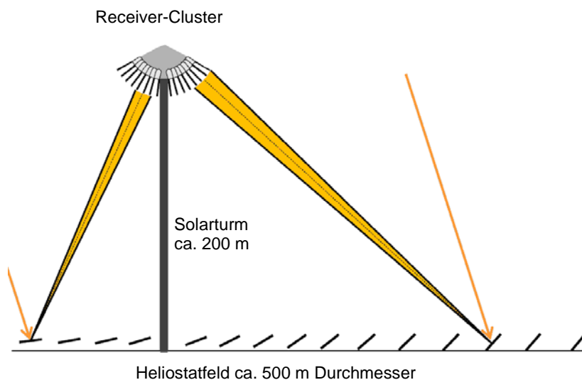
Abbildung 5: 50-MW-Kraftwerk-Modell «Facettenauge-Solarturm-Modell» für eine 50-MW-Kraftwerkanlage. 500 Receiver werden von Heliostaten im Umfeld von 500 m angestrahlt.
